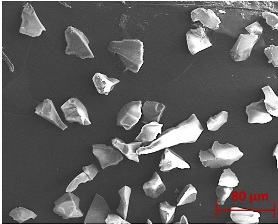
Elektronenmikroskopische Aufnahmen von Makrospec®50 – Granulat
